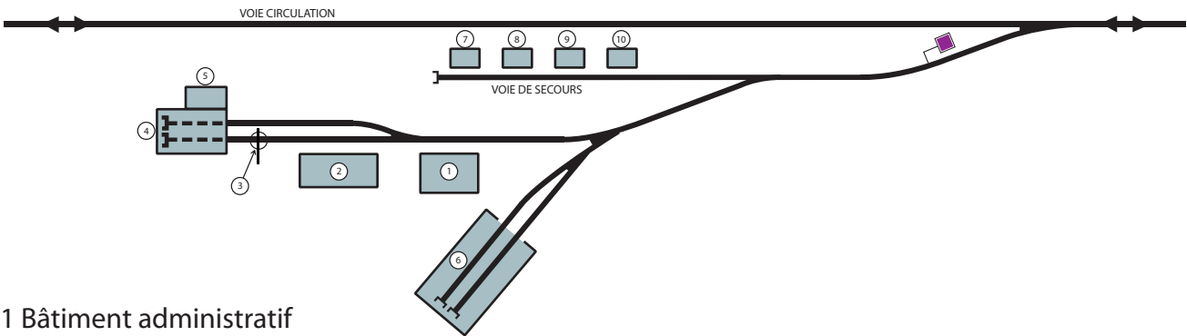
Fig. 63 – Schéma type d'un chantier de district.
